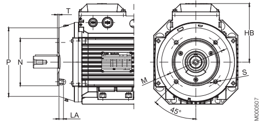
Flange-mounted motor, small flange; IM B14 (IM 3601)
