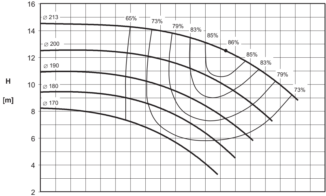
ENR4 100-200 MEI > 0.40
