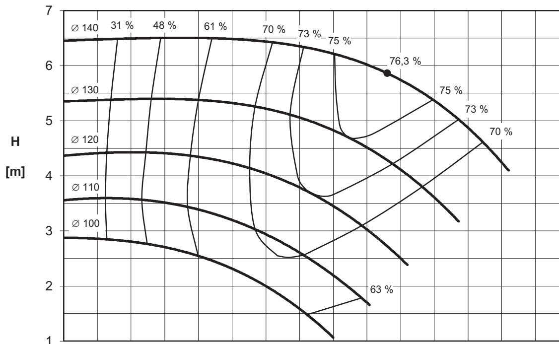
ENR4 50-125 MEI > 0.40
