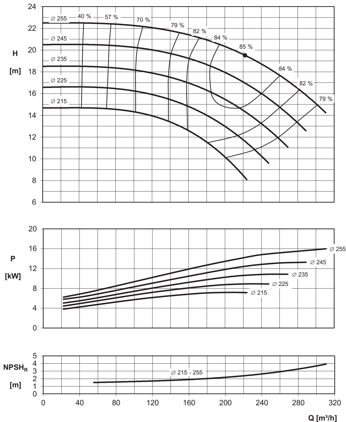
ENR4 125-250 MEI > 0.40
