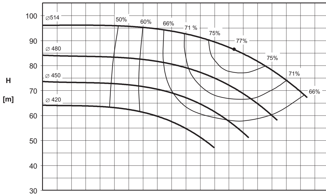
ENR4 150-500 MEI > 0.40
