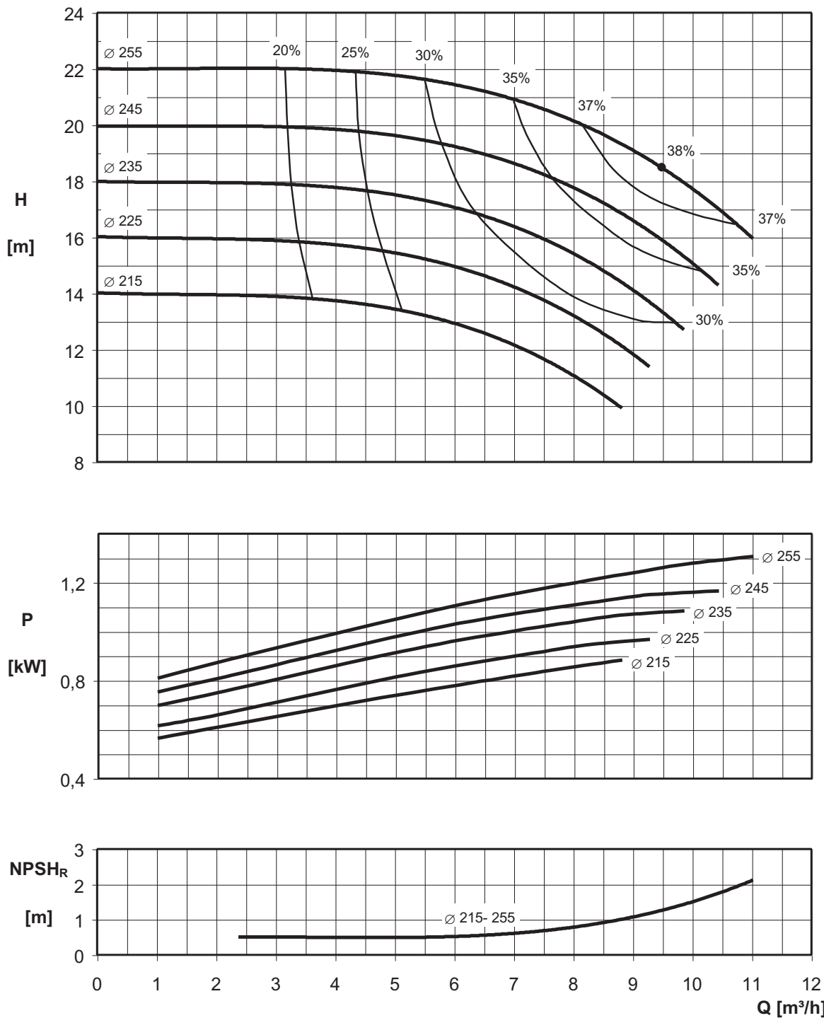
ENR4 32-250 MEI > 0.40
