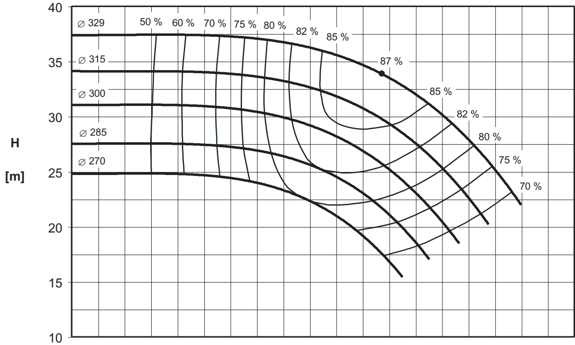
ENR4 125-315 MEI > 0.40
