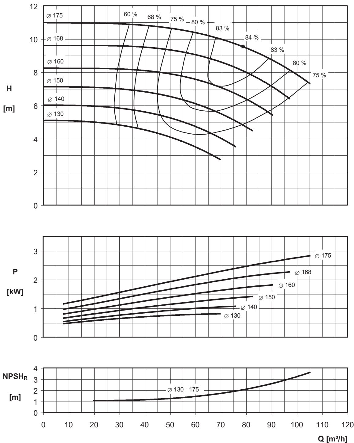
ENR4 80-160 MEI > 0.40
