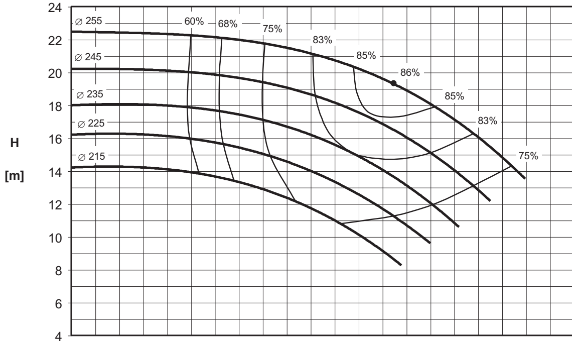
ENR4 100-250 MEI > 0.40
