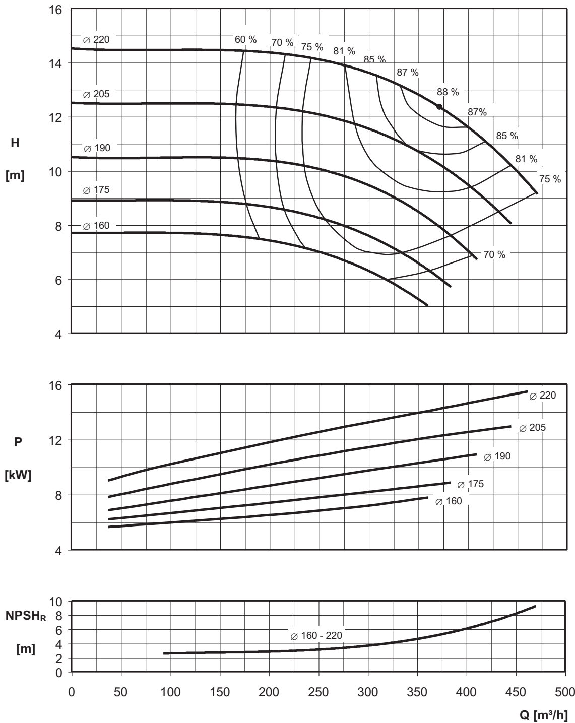
ENR4 150-200 MEI > 0.40
