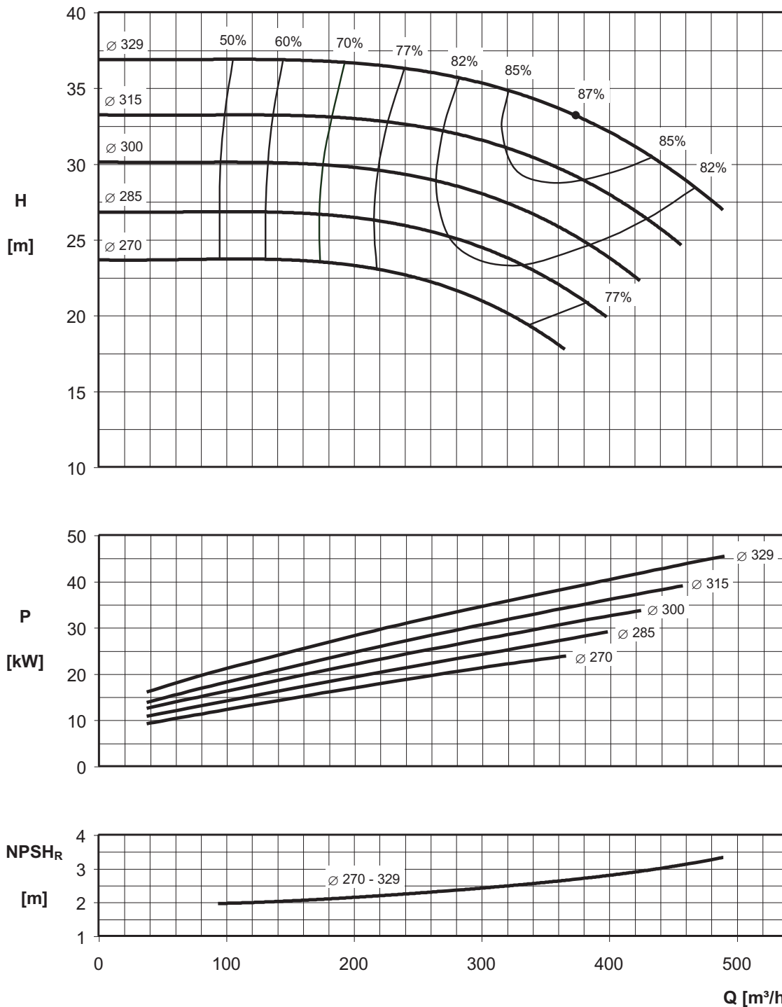
ENR4 150-315 MEI > 0.40
