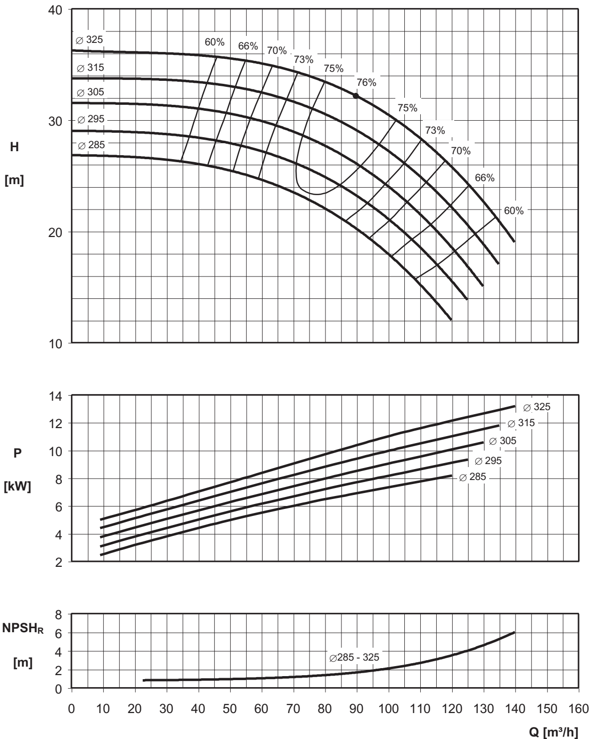
ENR4 80-315 MEI > 0.40
