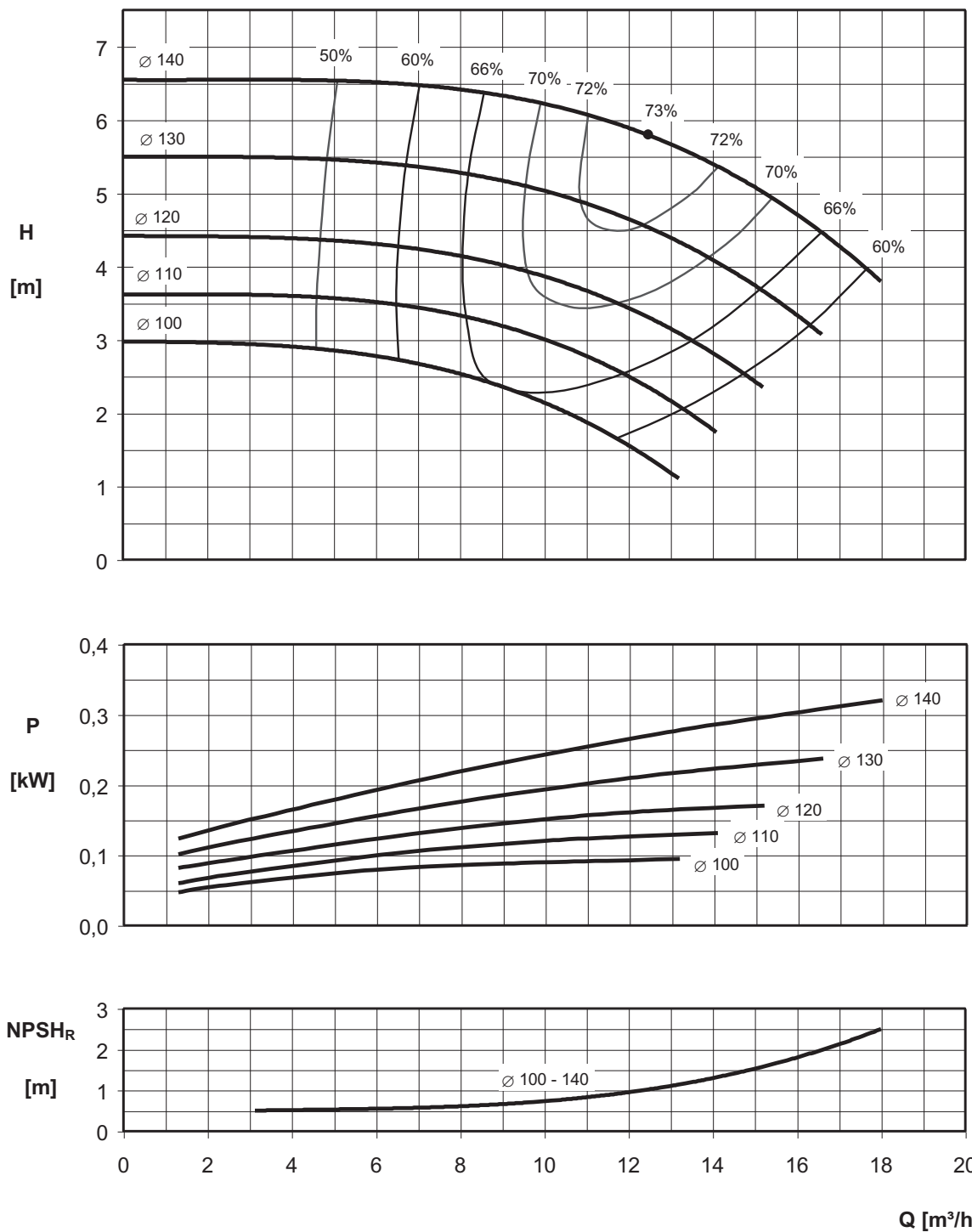
ENR4 40-125 MEI > 0.40
