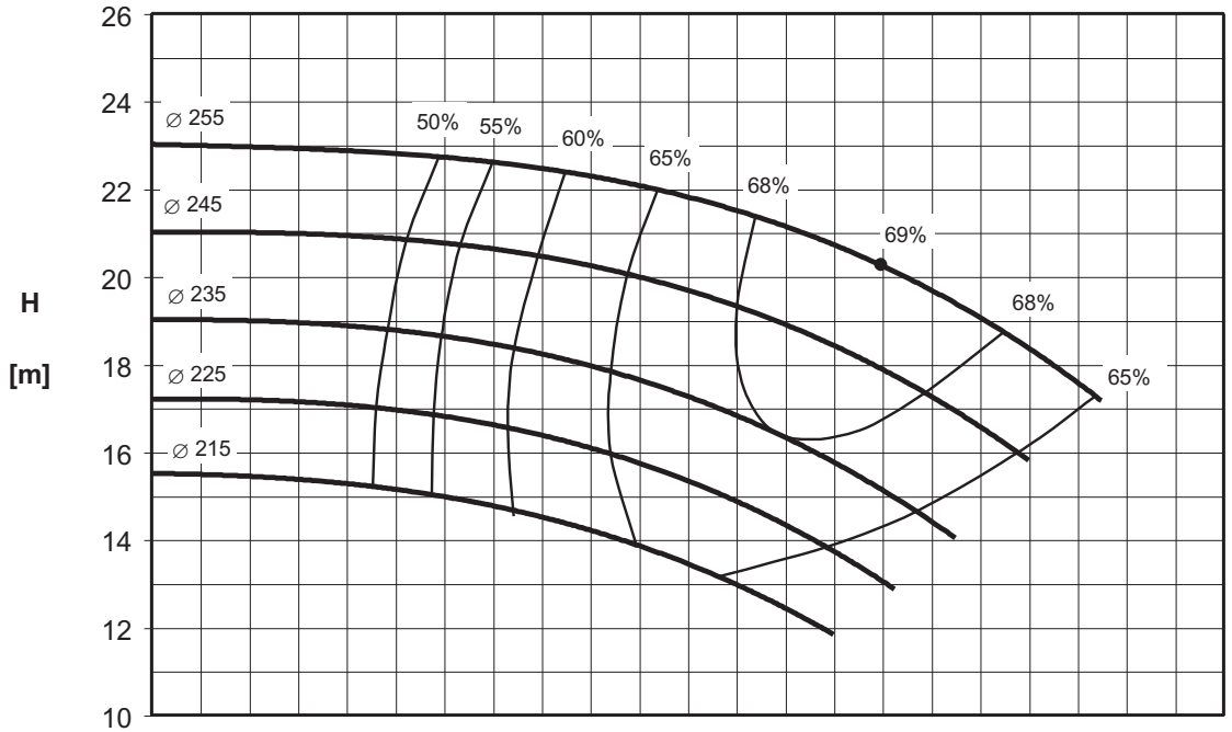
ENR4 50-250 MEI > 0.40
