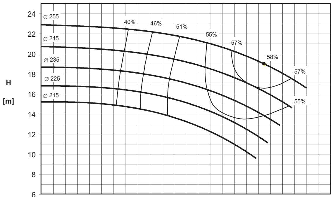
ENR4 40-250 MEI > 0.40
