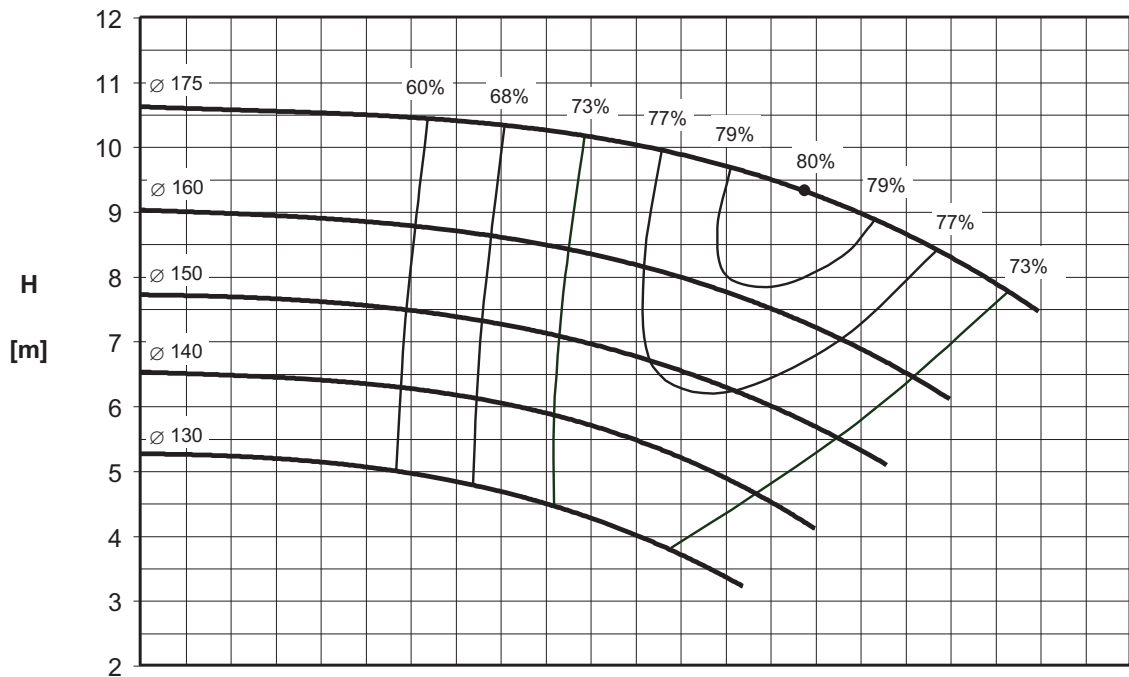
ENR4 50-160 MEI > 0.40
