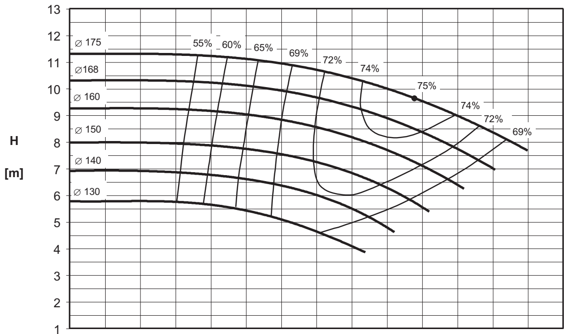
ENR4 40-160 MEI > 0.40
