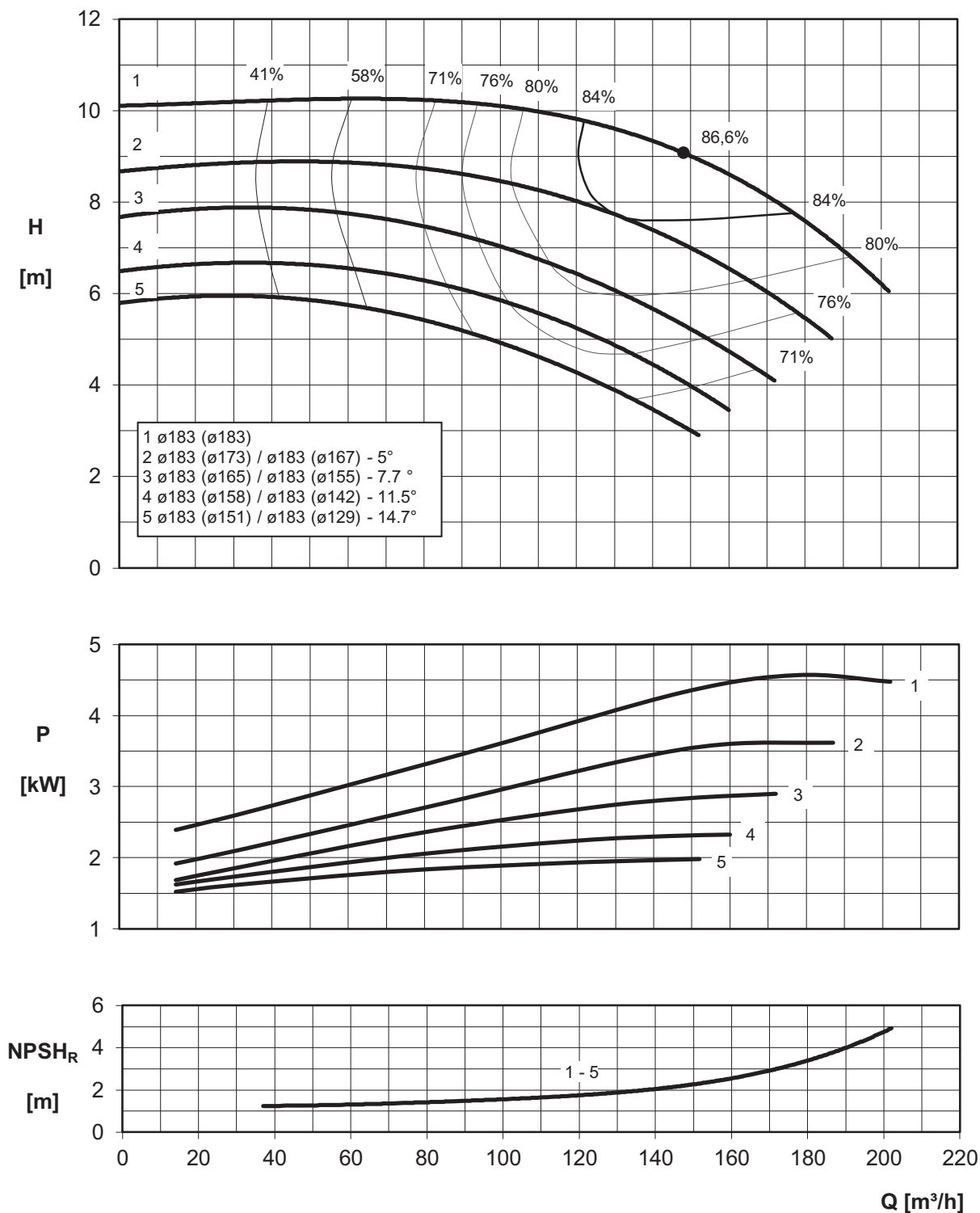
ENR4 100-160 MEI > 0.40
