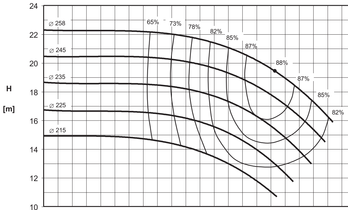
ENR4 150-250 MEI > 0.40
