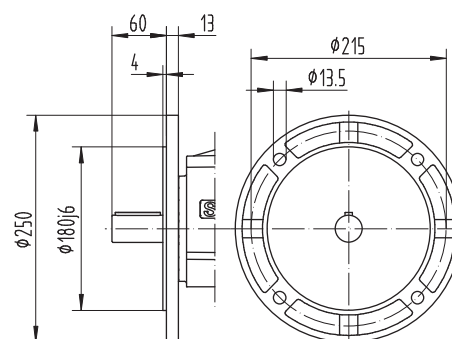
III Ø250
