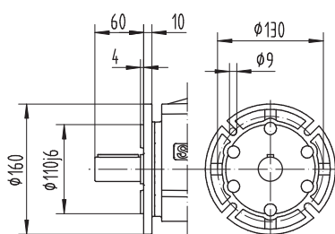
I Ø160
