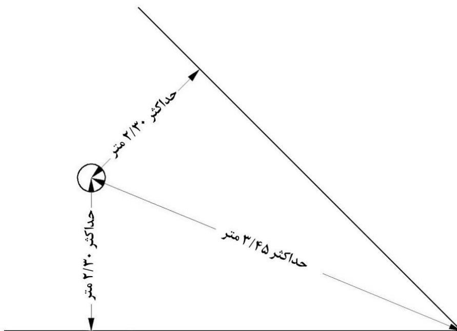
شکل ۴-۴-۱۱- حداکثر فاصله اسپرینکلر از کنج دیوار
