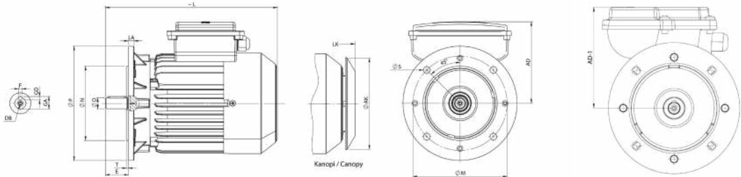
FLANGED MOTOR (TYPE “A” - IEC 60072-1) - B5, V1, V3
