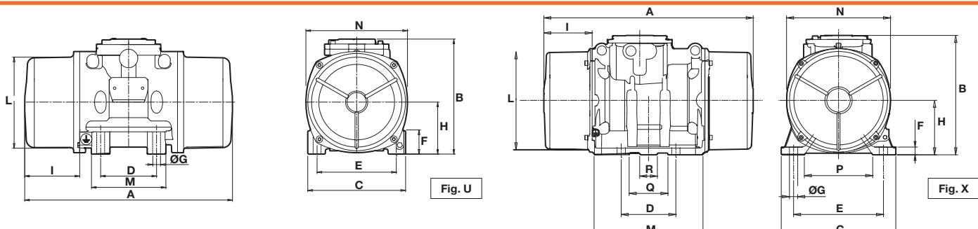
CARATTERISTICHE DIMENSIONALI (mm)
