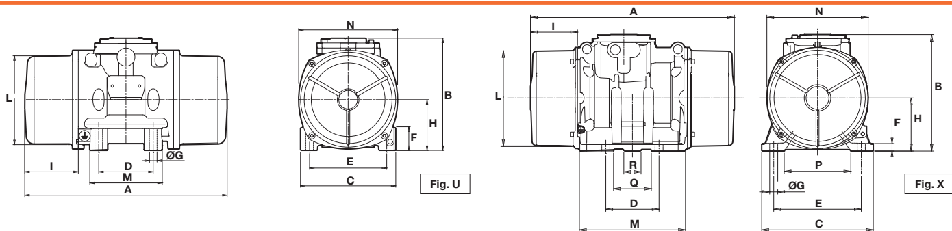
CARATTERISTICHE DIMENSIONALI (mm)
