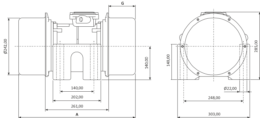
Gövde Ölçüleri - Overall Dimensions (mm)
