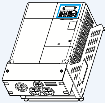
Drive + Conduit
