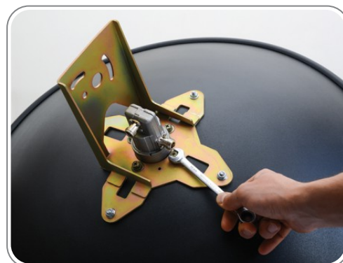
۷- نحوه بستن پیچ فید و پیچ و مهره‌های پایه
