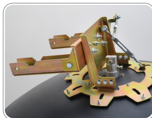
۱۱ - نحوه نصب کرپی ها جهت اتصال آنتن به دکل
