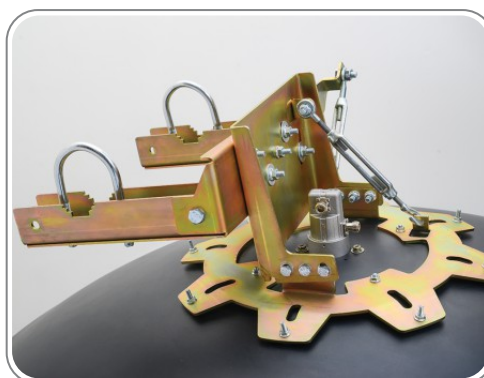
۱۰ - نحوه قرار گرفتن متعلقات آنتن
