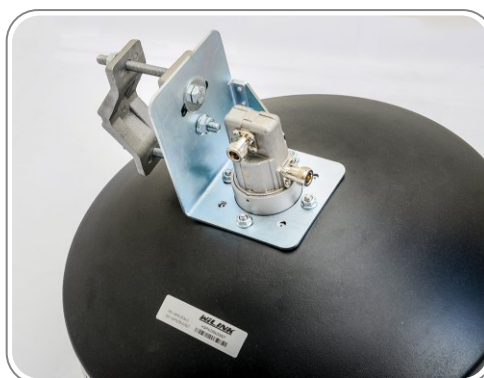
۱۱ - نمایی از یک آنتن موتناژ شده کامل
