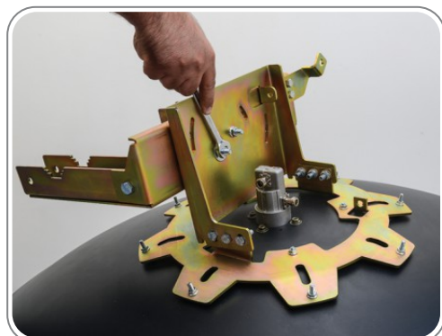
۳- نحوه قرار دادن پایه خرنجی در کنار پایه اصلی
