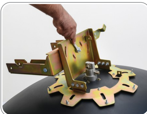
۴- محل نصب پیچ رابط پایه خرنجی به پایه
