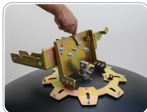
۸- نصب مهرکش دوم جهت حرکت افقی سر آنتن دیش به صورت میلیمتری (Fine Tune)
