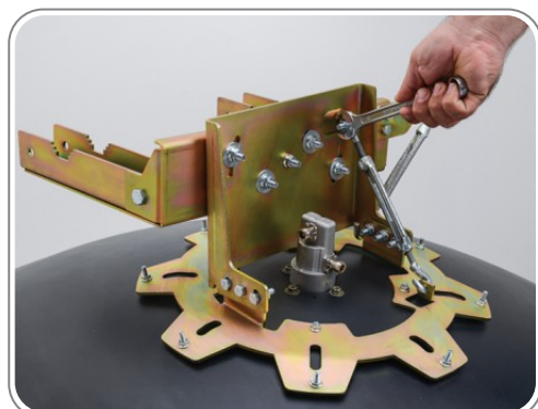
۶- نحوه محکم کردن پیچ و مهره متحرک
