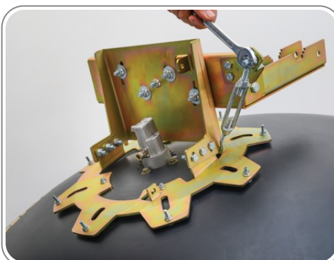
۷- نصب مهرکش اول جهت حرکت عمودی سر آنتن دیش به صورت میلیمتری (Fine Tune)
