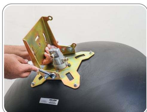
۵ - نحوه بستن پیچ پایه ستاره‌ای
