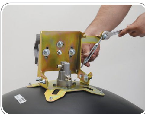
۱۴ - نصب مهارکش اول جهت حرکت عمودی سر آنتن به صورت میلیمتری (Fine Tune)
