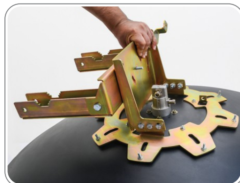
۵- محکم کردن مهره پیچ رابط پایه خرنجی به پایه
