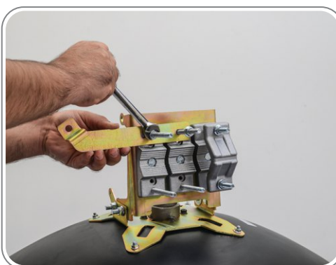
۱۱ - نحوه نصب قطعه مخصوص اتصال مهارکش
