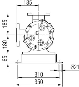
YKUYF 2½"
