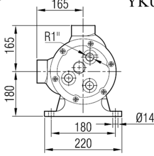
YKU 2½"
