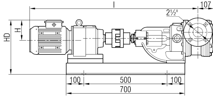
YKU 2½"
