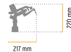
Dimensions / Abmessungen
