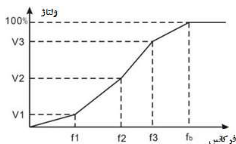
نمودار ۹-۶ تنظیم نمودار منحنی V/F
