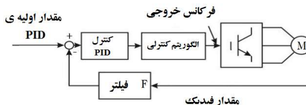
شکل ۶-۲۲ دیاگرام کنترل PID
