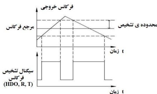
شکل ۶-۲۰ نمودار تشخیص فرکانس
