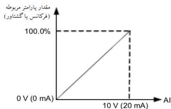
شکل ۶-۱۳ رابطه بین AI و تنظیم مربوطه
