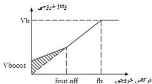
شکل ۸-۶ تقویت گشتاور به صورت دستی
