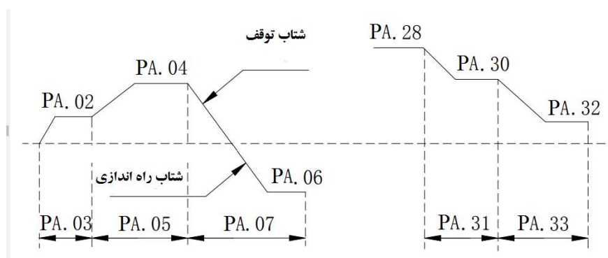
شکل ۲۴-۶ نمودار عملکرد Simple PLC
