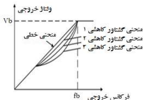
شکل ۶-۷ منحنی V/F
