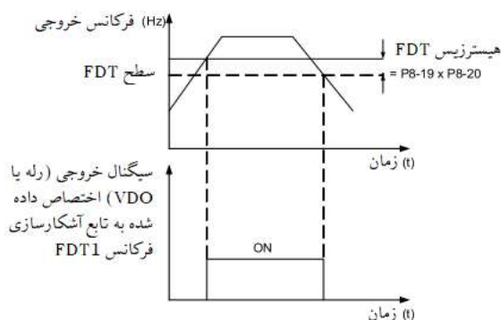
نمودار ۶-۱۹ سطح FDT و نمودار تاخیر
