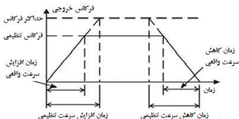
شکل ۶.۱ افزایش و کاهش سرعت
