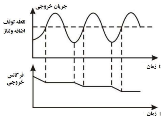
شکل ۳۲-۶: منحنی حفاظت از اضافه ولتاژ
