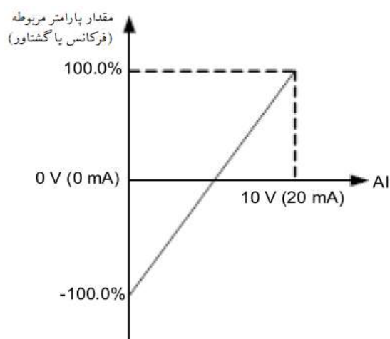
شکل ۶-۱۳ رابطه بین AI و تنظیم مربوطه
