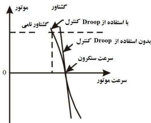
شکل ۲۱-۶ نمودار کنترل افتادگی
