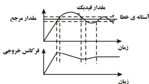
شکل ۲۳-۶ رابطه میان فرکانس خروجی و آستانه بایاس
