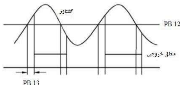
شکل ۳۳-۶ تابع کنترل اضافه گشتاور
