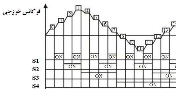
شکل ۲۹-۶ نمودار عملکرد حالت چند سرعت
