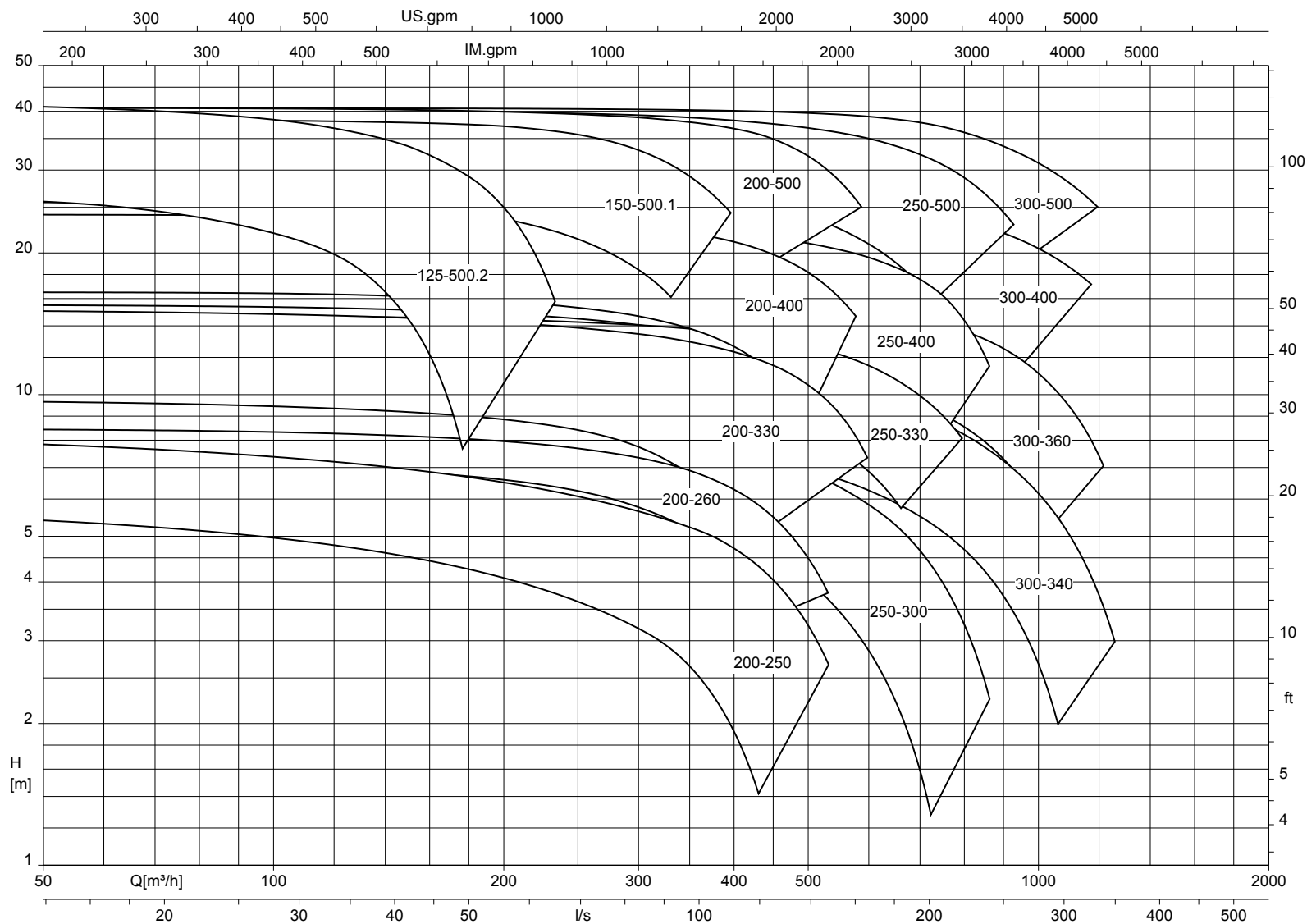
Etanorm-R, n = 960 rpm
