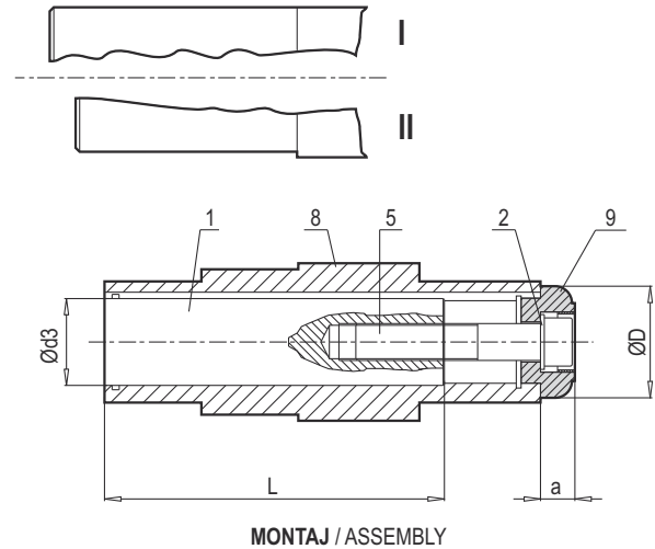
MONTAJ / ASSEMBLY
