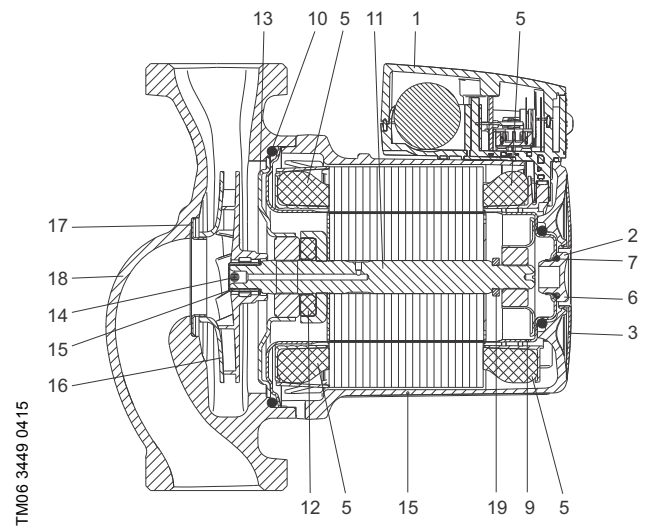
Fig. 7 UPS xx-100
