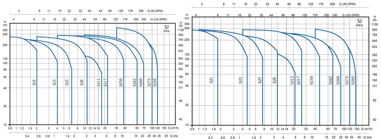
جدول ارتفاع و آبدی سری SJ استریم چین
