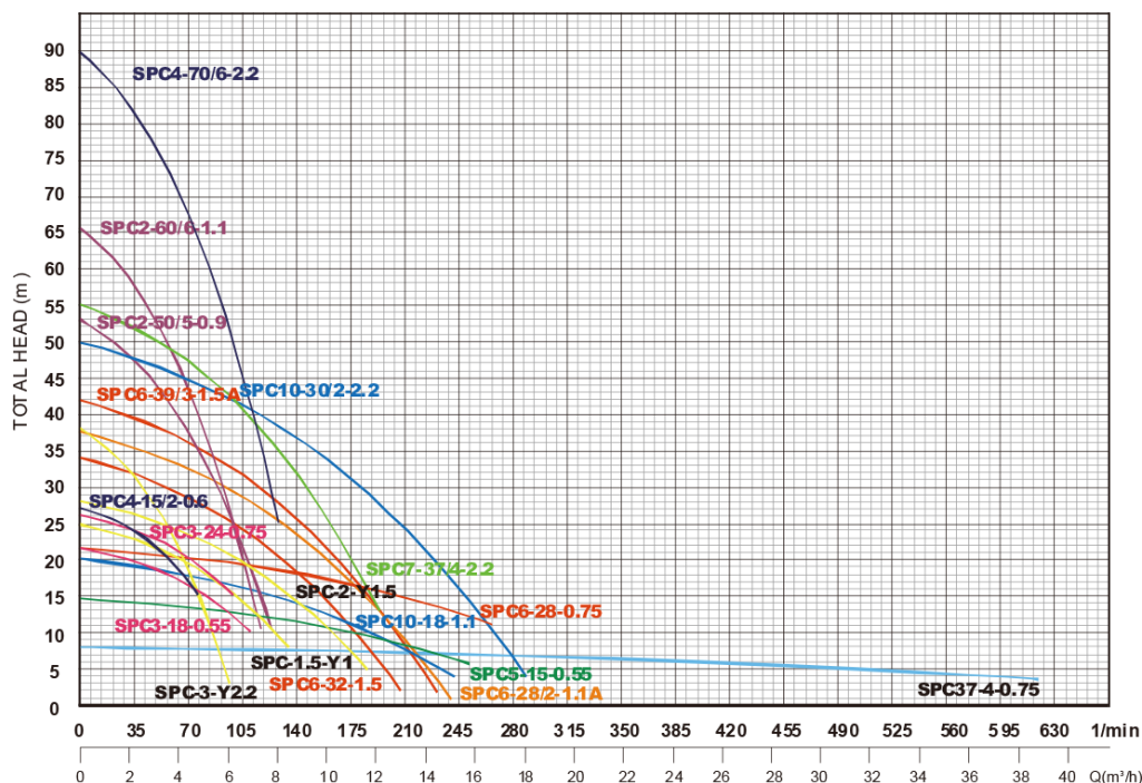
جدول ارتفاع و آبدهی الکتریمپ خودمکش سری SPC استریم چین
