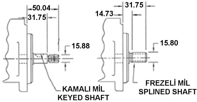
Opsiyonel Mil Bağlantıları Optional Shaft
