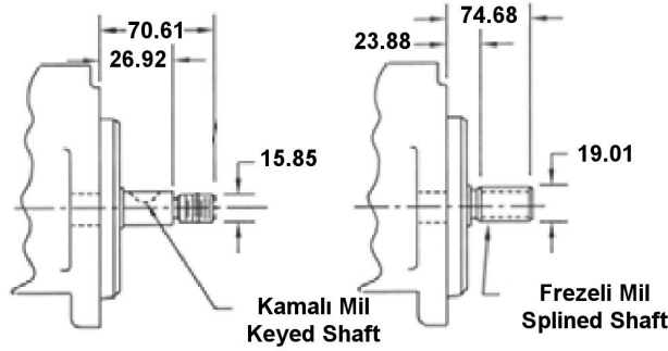
Opsiyonel Mil Bağlantıları Optional Shaft
